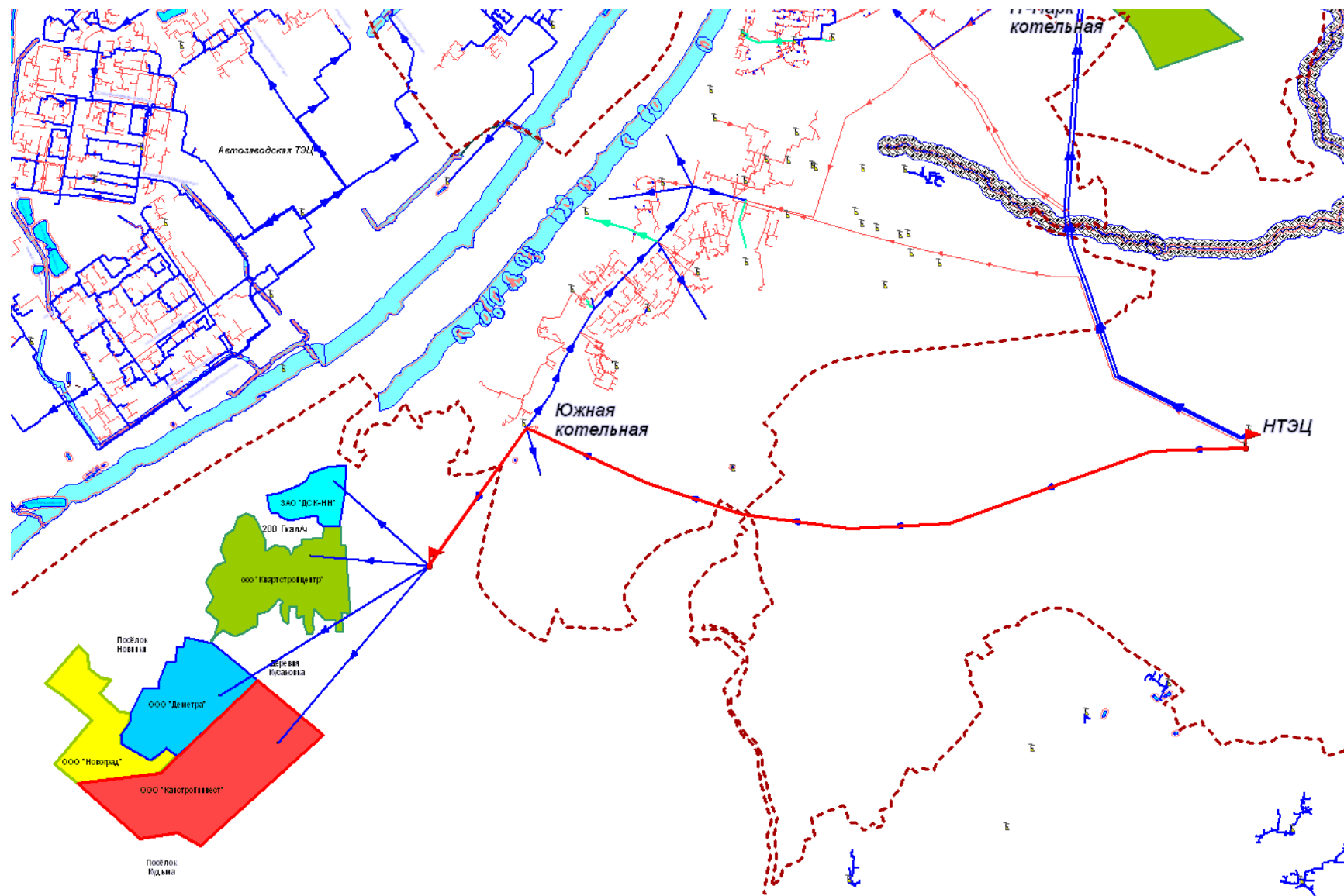
Рисунок 2.15 – Трасса от НТЭЦ по Южной т/м через Южную котельную до Новинок
