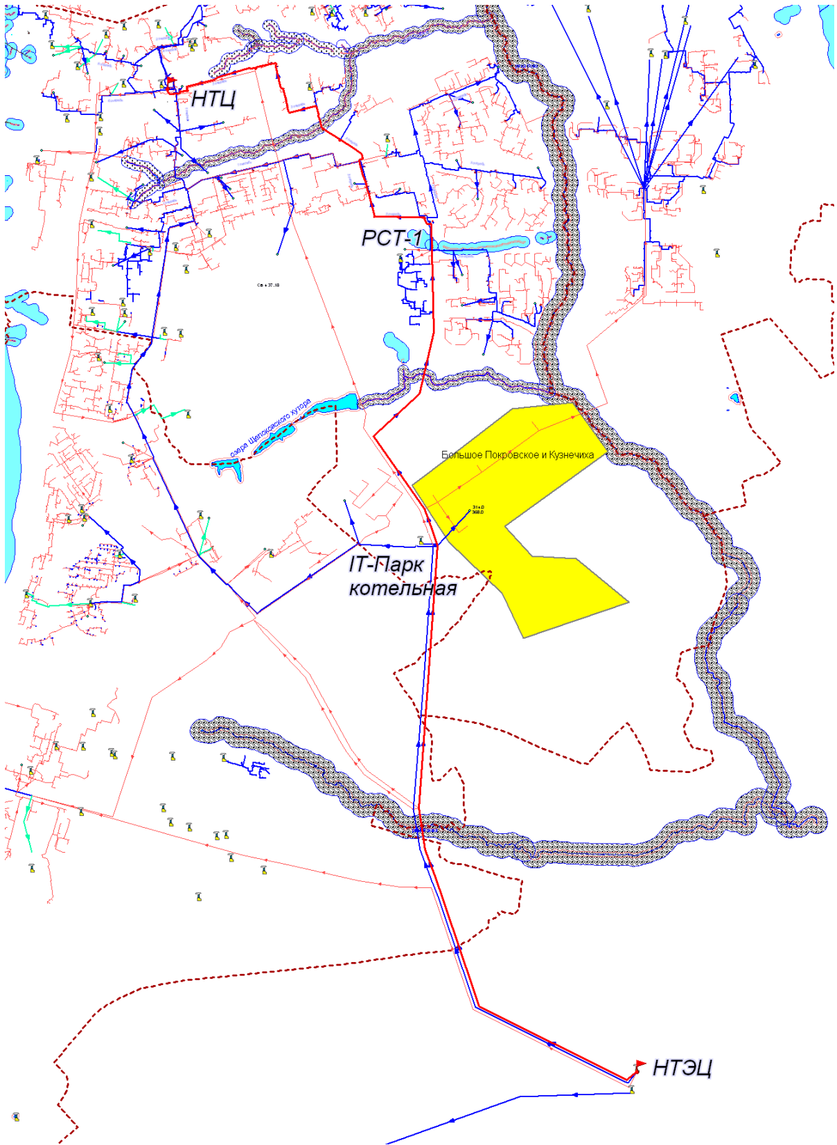
Рисунок 2.9 –Трасса от НПТЭЦ через РСТ-1 по т/м «3 очередь» до HTЦ
