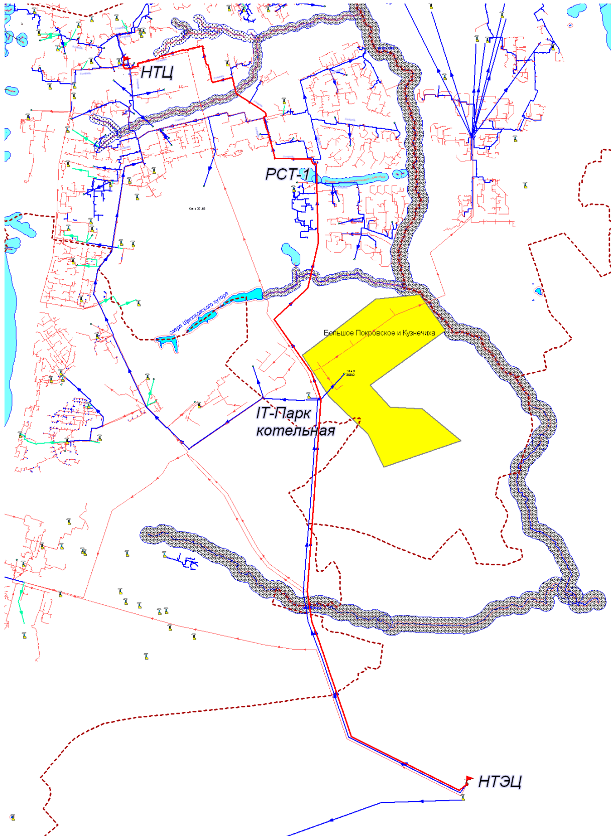
Рисунок 2.2 – Трасса от НТЭЦ через котельную ИТ-Парка, через РСТ-1 по т/м «3 очередь» до НТЦ
