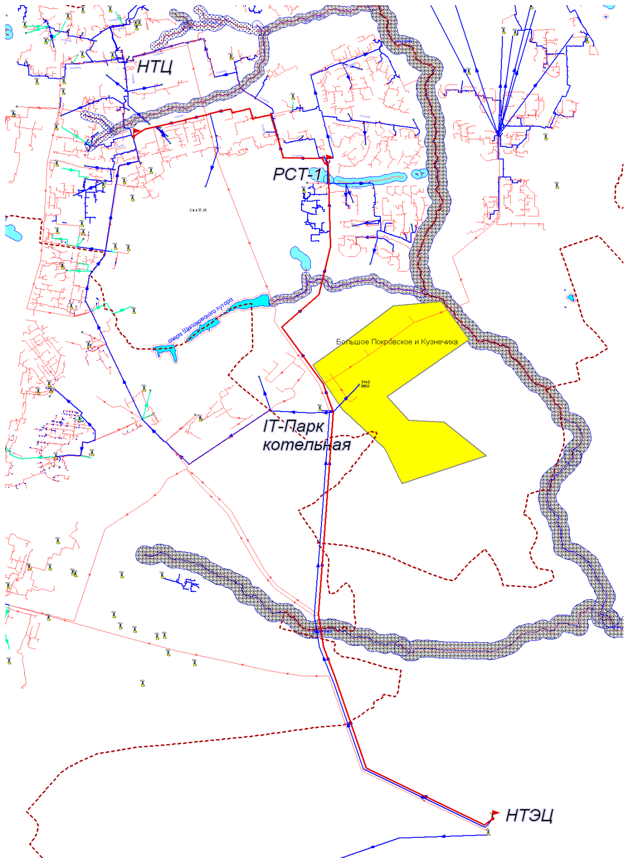
Рисунок 2.4 –Трасса от НГТЭЦ через котельную IT-Парка, РСТ-1 по т/м «1 очередь» до ТК-112
